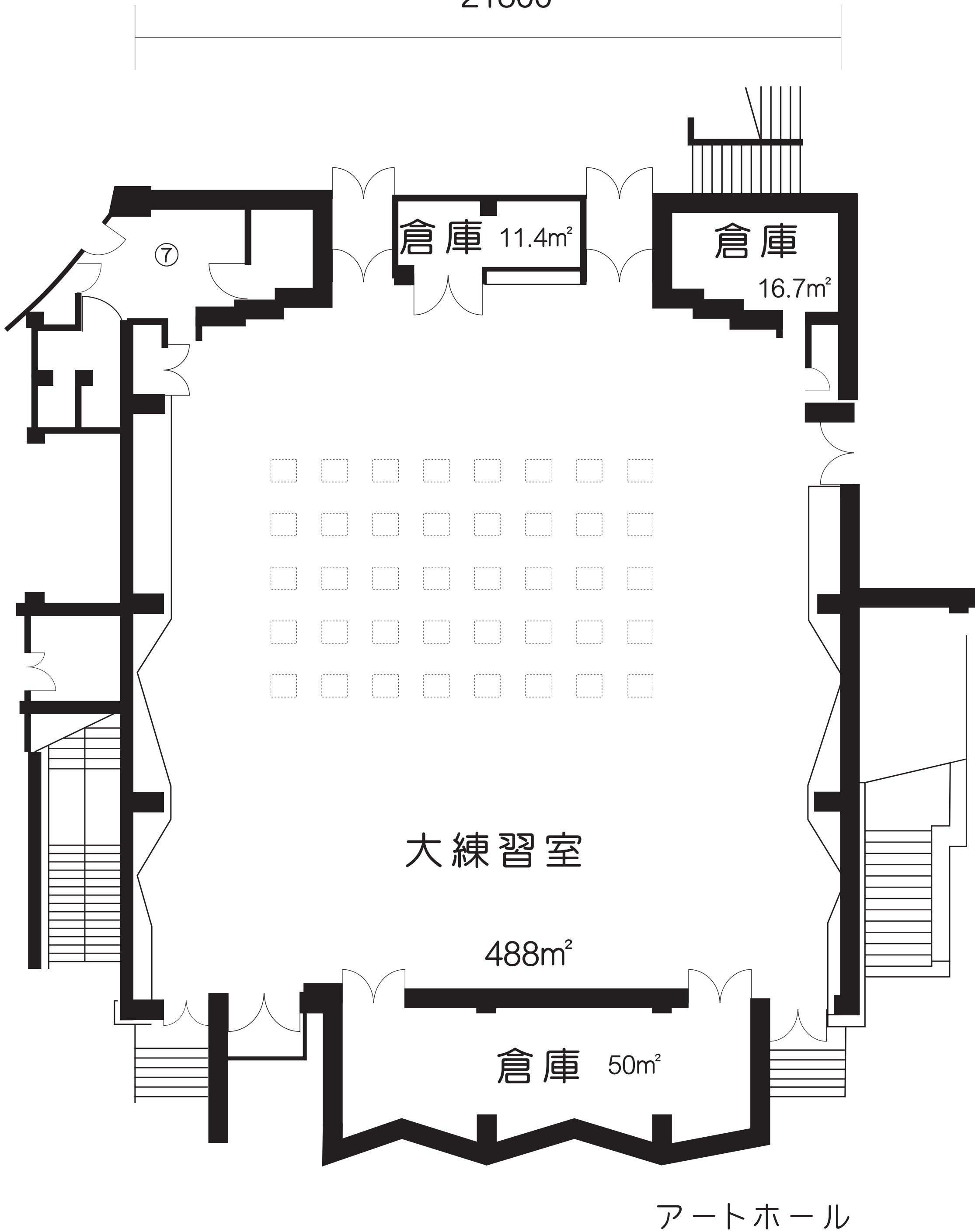
1階大練習室平面図 1/100
